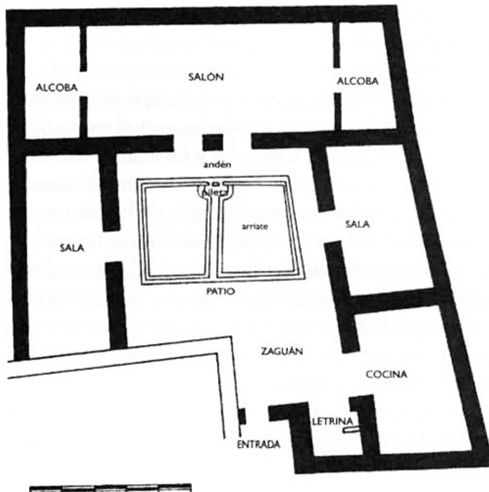
Planta de una casa de época califal. (Según Fernández y López, 1993)
